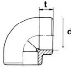
90° ELBOW 0102
